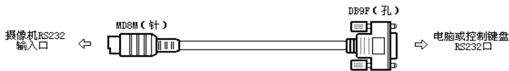
图 2-3 RS-232 接口示意图
